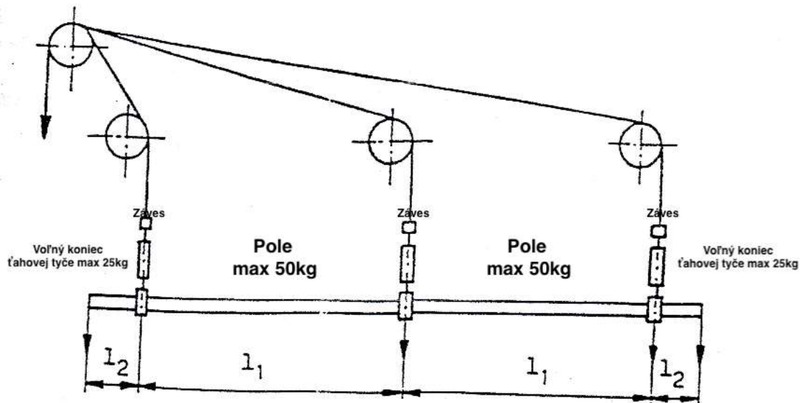
l1 - vzdialenosť medzi závesmi l2 - dĺžka voľného konca ťahovej tyče
