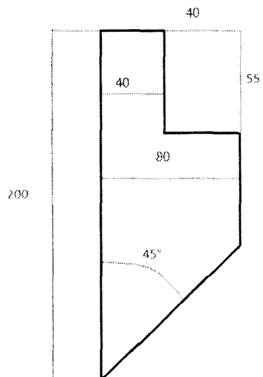
Obrázok č.2 – Gumo-textilný brit s úkosom a s kopýtkom na uchytienie
