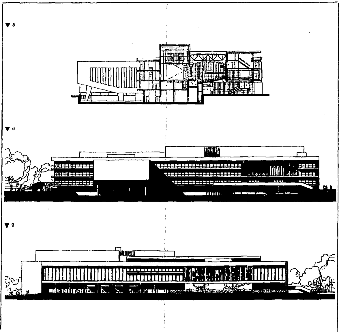
REZY A POHLÁDY pre znázornenie výškových úrovní strešnej roviny objektu.
