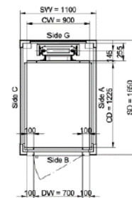
FLOOR 0 Scale: 1:30
