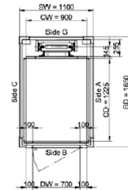
FLOOR 1 Scale: 1:30
