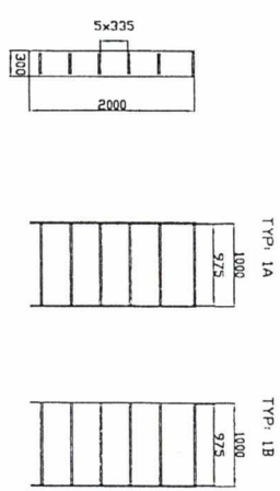
STABILNÉ POLICOVÉ REGÁLE - JEDNOSTRANNÝ PRÍSTUP - Šírka: 300 mm
