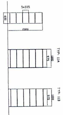
STABILNÉ POLICOVÉ REGALE - OBOUSTRANNÝ PRÍSTUP - ŠÍRKA 600 mm
