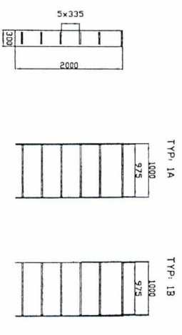
STABILNÉ POLICOVÉ REGALE - JEDNOSTRANNÝ PRÍSTUP - šírka: 300 mm
