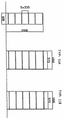
STABILNÉ POLICOVÉ REGALE - OBOJSTRANNÝ PRÍSTUP - šírka 600 mm
