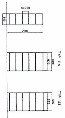
STABILNÉ POUICOVÉ REGÁLE - OBOUSTRANNÝ PRÍSTUP - ŠÍRKA 600 mm
