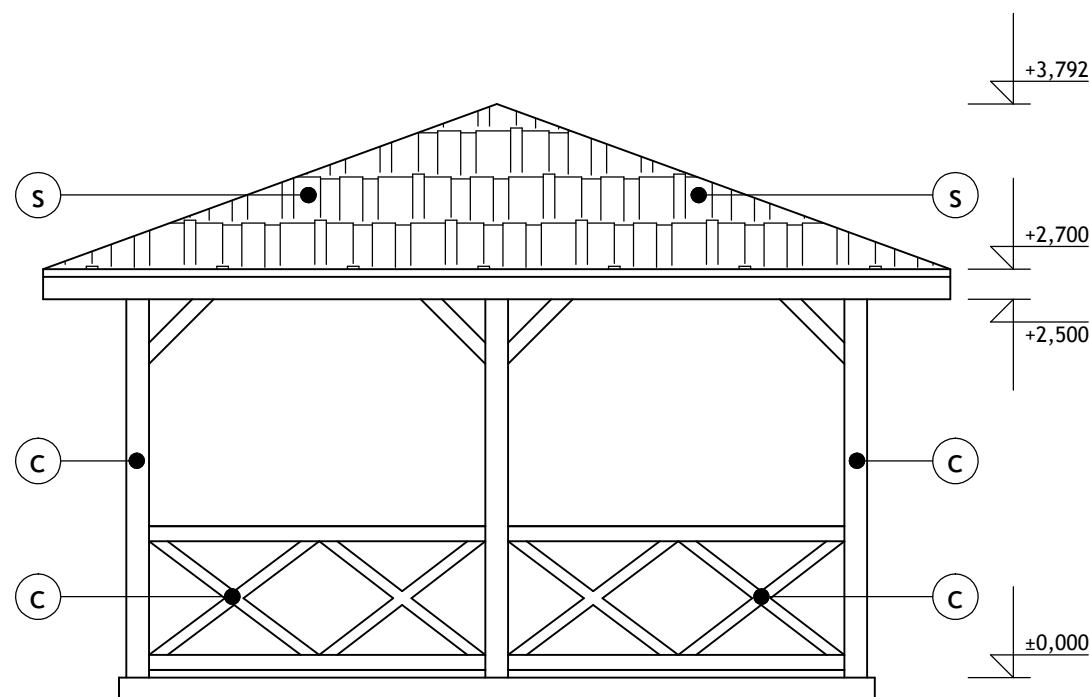
POHLAD VÝCHODNÝ
