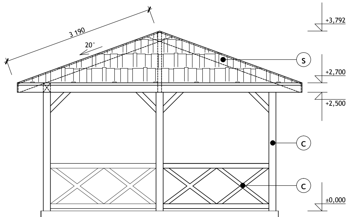
POHLAD JUŽNÝ
