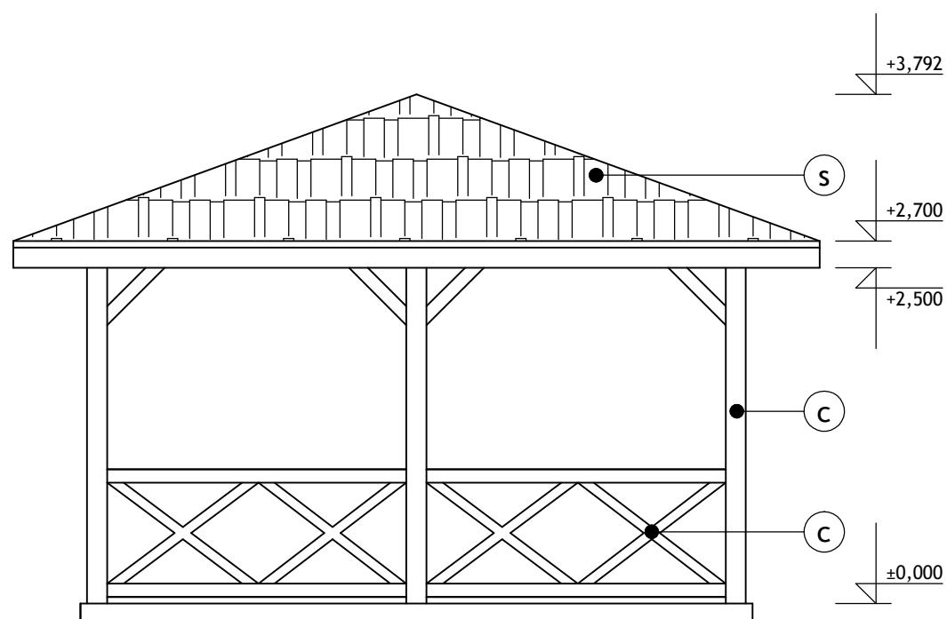
POHLAD ZÁPADNÝ
