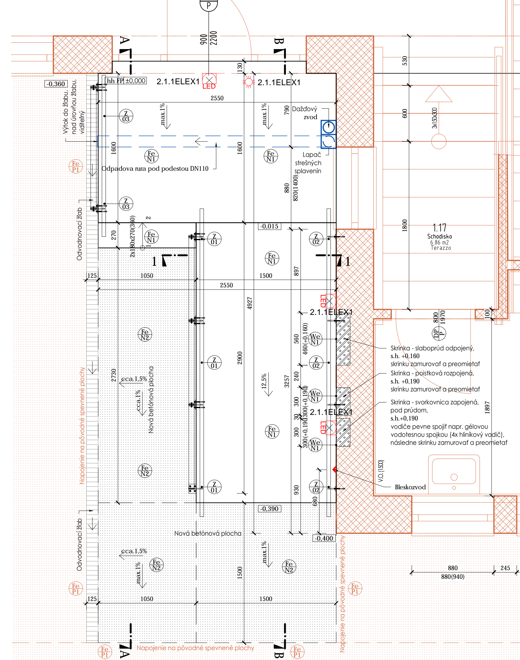
PŌDORYS RAMPY, m1:25
