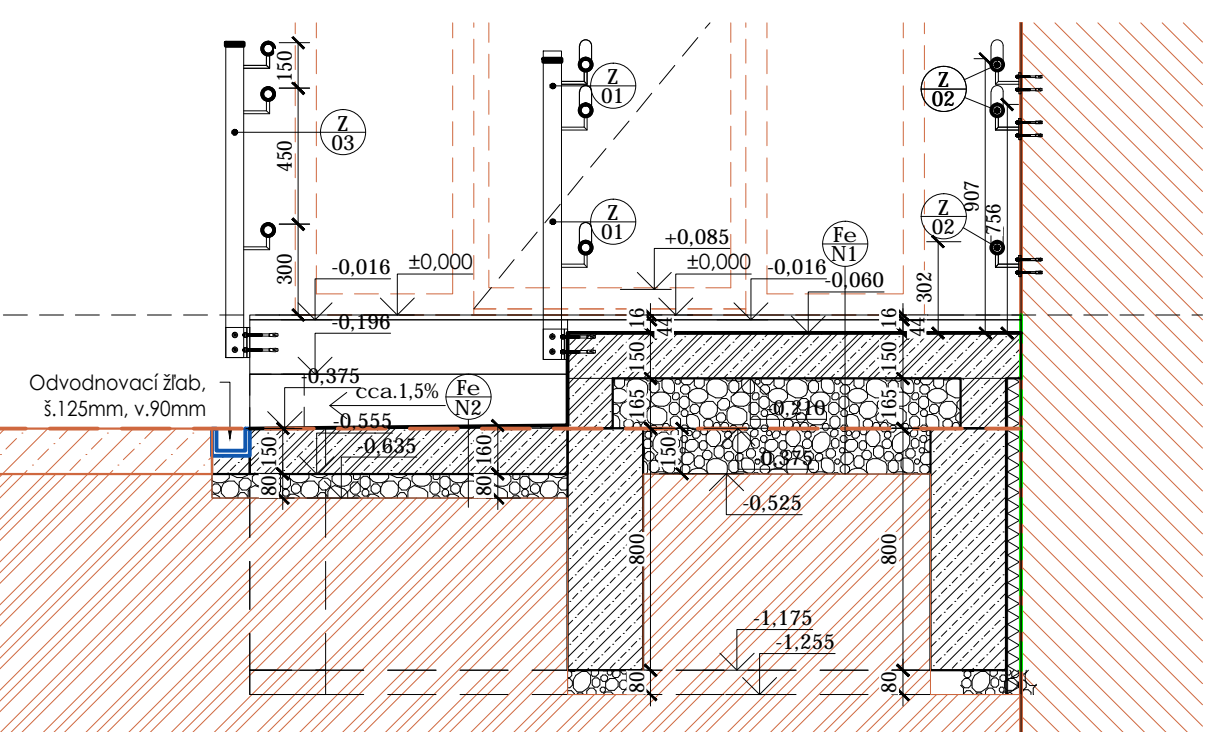
REZ 1-1, m1:25
