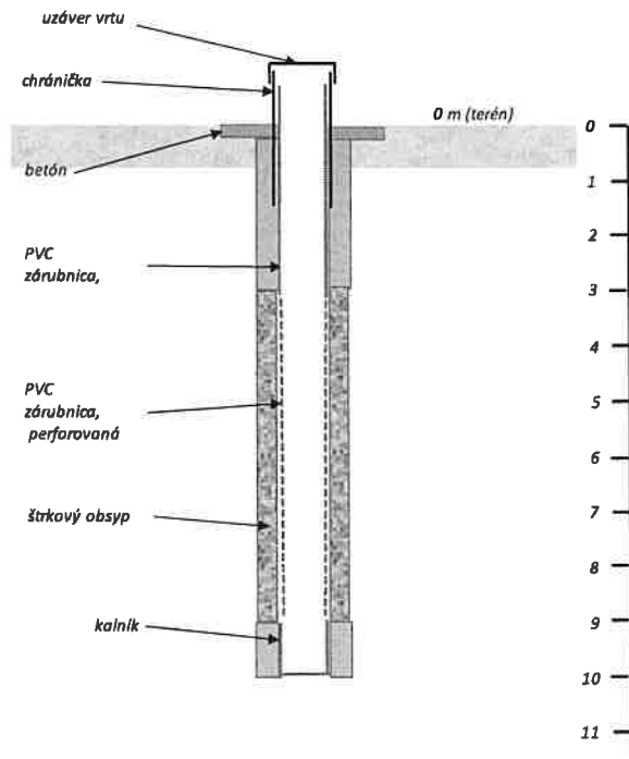
Obr. 1 Schéma zabudovania prieskumných monitorovacích vrtov
