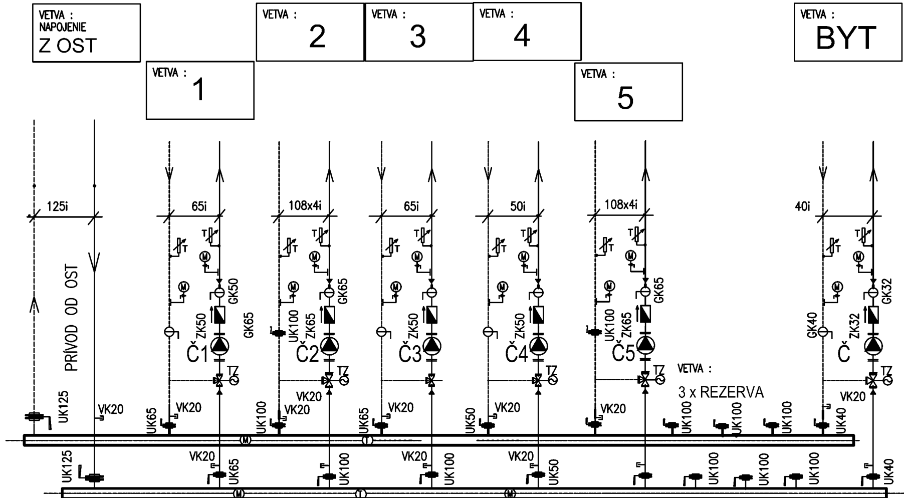
DOM KULTÚRY DÚBRAVKA, Saratovská 2 SCHÉMA ZAPOJENIA VYKUROVACÍCH VETIEV
