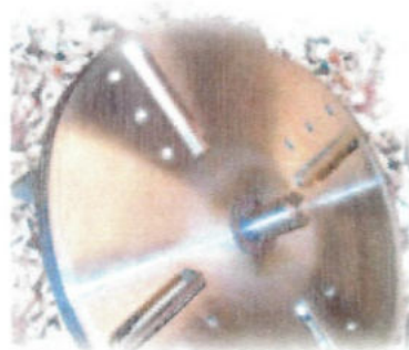
Rezací disk so 4 nožmi
