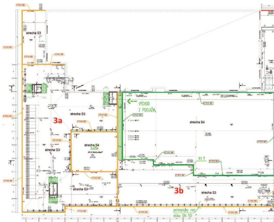
Pozn. Pôdorys strechy S3
