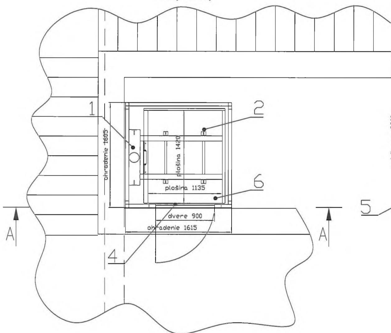
Pôdorys šachty
