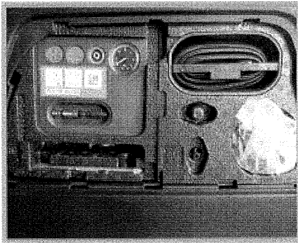
Funkčná súprava na opravu pneumatík
