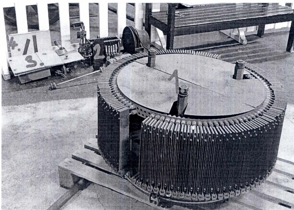
Obr.1 Zrýchľovač z električkového vozňa ČKD Tatra T3SUCS s príslušenstvom: (1. Zrýchľovač s ovládacím motorom, 2. pedále, 3. skrinka hlavného vypínača, 4. tabuľka)
