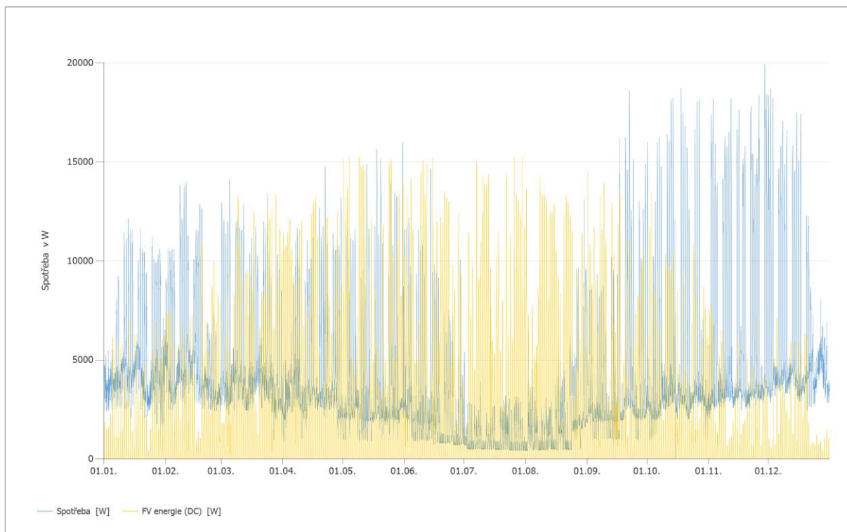
Obrázok: Spotreba EE na OM v porovnaní s výrobou EE z FVE
