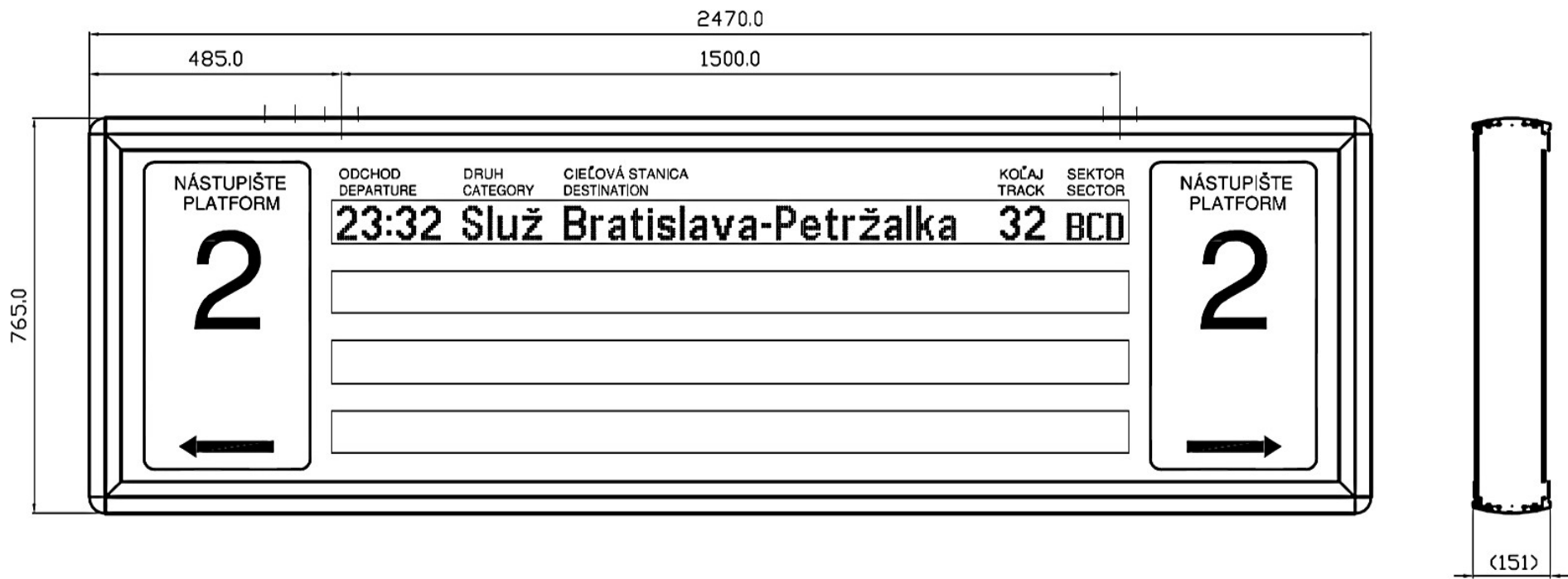
Obr. Podchodová tabuľa TDR 76-16/320x4 RG L55
