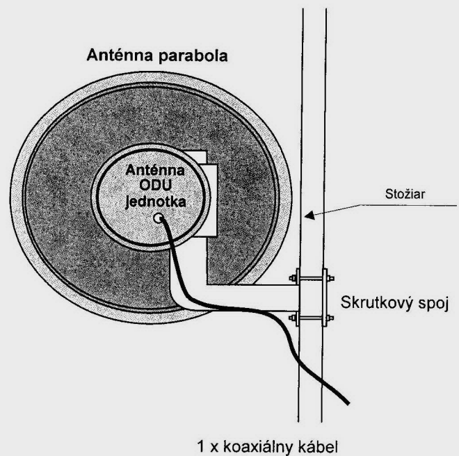
Antény stožiar typu L - pohľad zo zady
