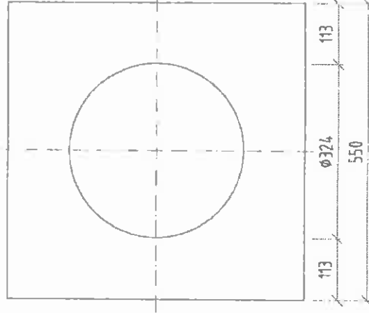
Poz. 3 / P.12x550-550 /
