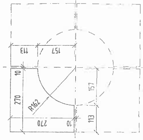
Poz. 4 / P.12x270-270 /
