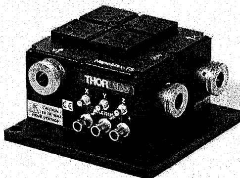
Obr. b) Ilustračná fotografia dodávaného Systému pre polohovanie PCF vlákien MAX311/M.
